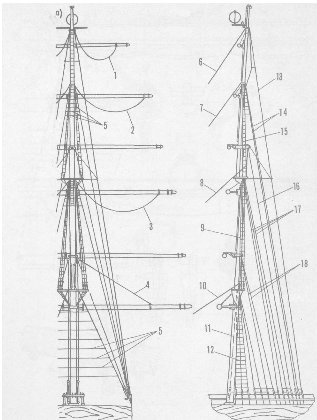
Рис. 30. Стоячий такелаж: а — мачта с прямым вооружением;
