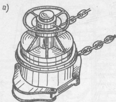
Рис. 6. Стопоры якорных цепей: а — ленточный шпильевой; б — палубный винтовой
