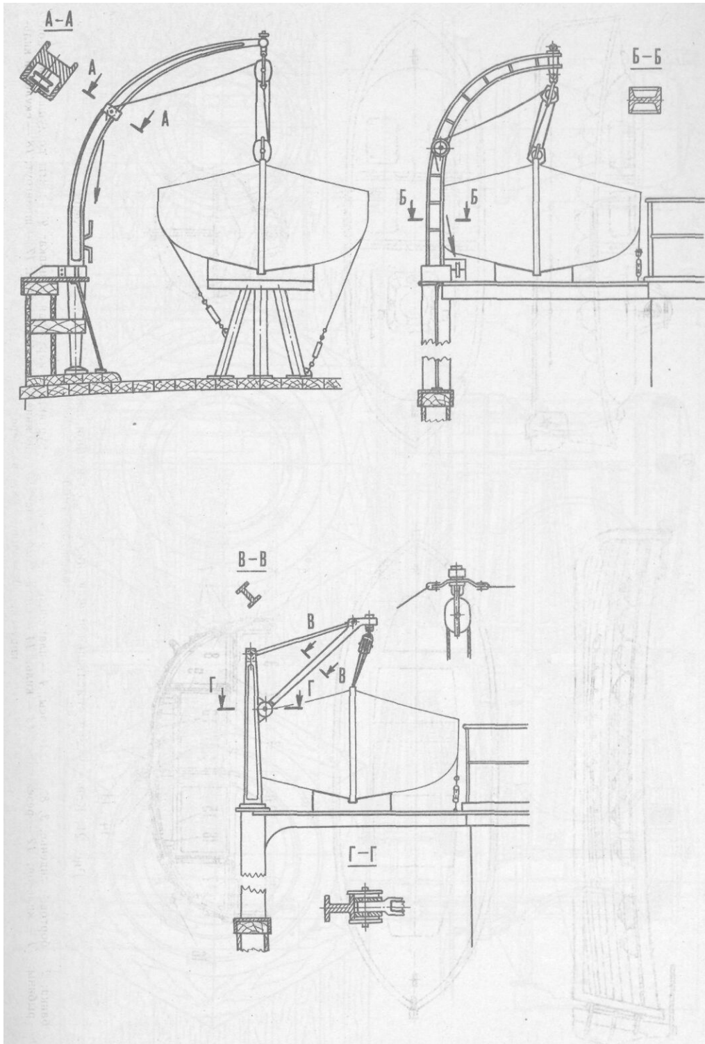
Рис. 22. Различные типы поворотных шлюпбалок
