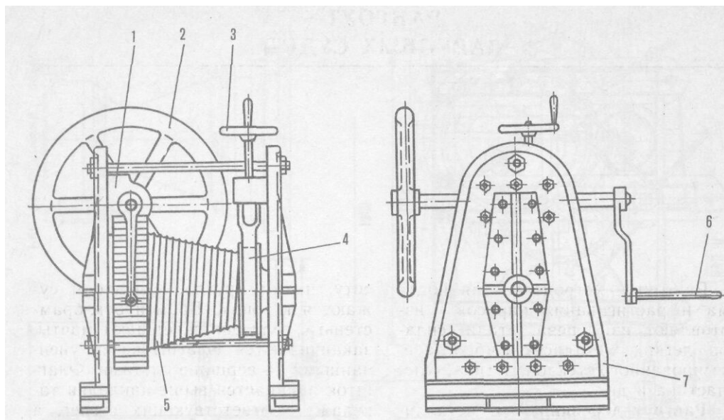
Рис. 25. Марсафальная лебедка
