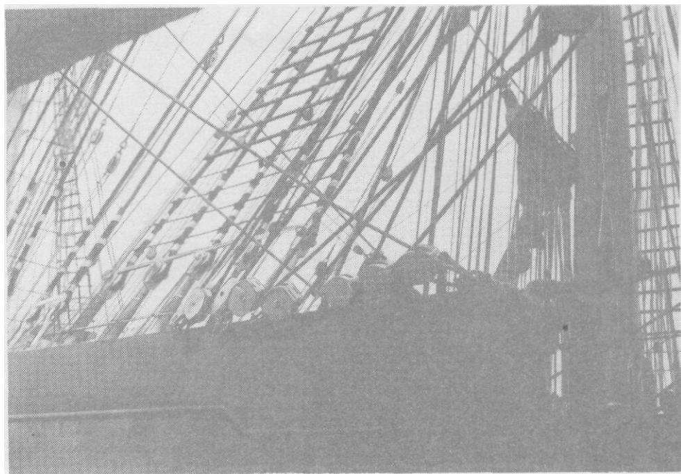
Рис. 64. Отводные брас-блоки
