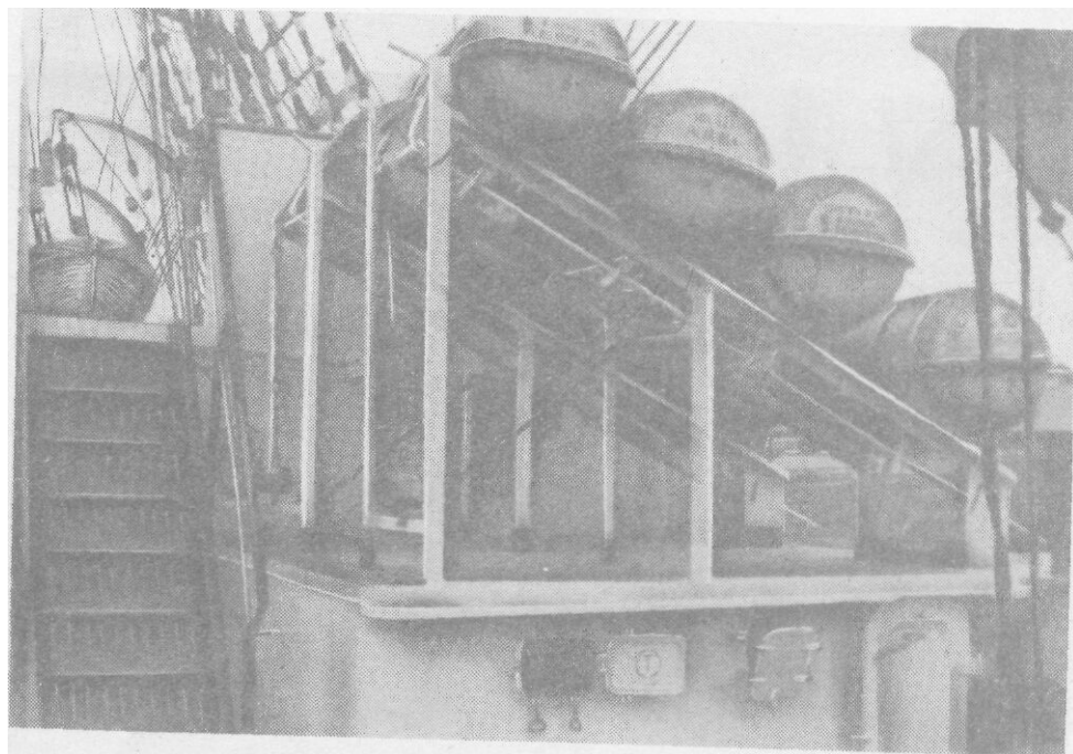
Рис. 51. Надувные спасательные плоты в контейнерах
