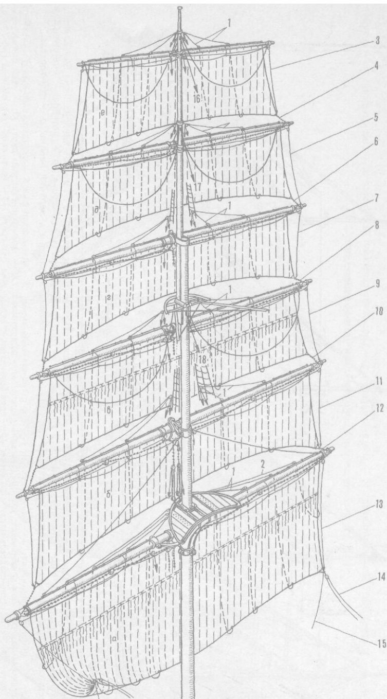
Рис. 37. Паруса и бегучий такелаж мачты с прямым вооружением:
