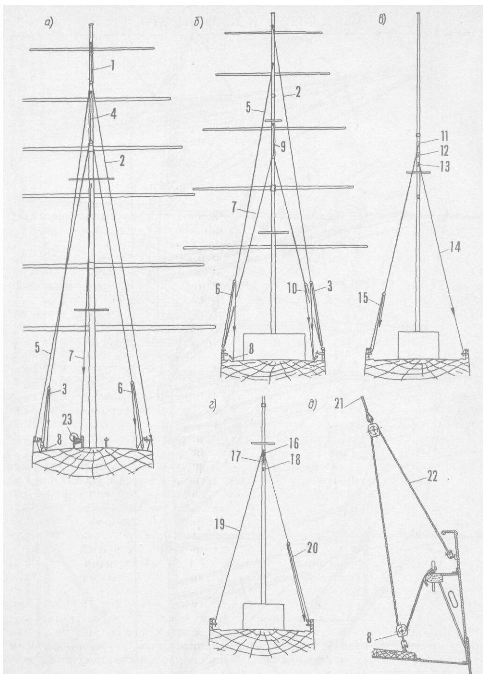
Рис. 33. Фалы реев, гафеля, стакселей и кливеров: а — мачта четырехмачтового барка; б — мачта трехмачтовой баркентины; в — дирик-фал и гафель-гардель гафелей мачт трехмачтовой баркентины; г, д — лопари стаксель (кливер)-фала
