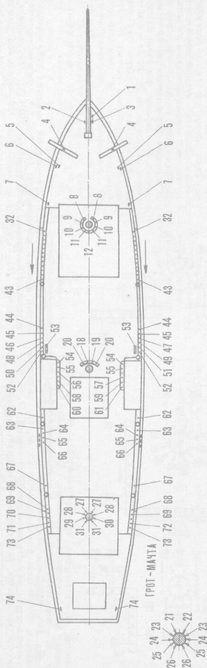
Рис. 43. План крепления снастей трехмачтовой баркентины.
