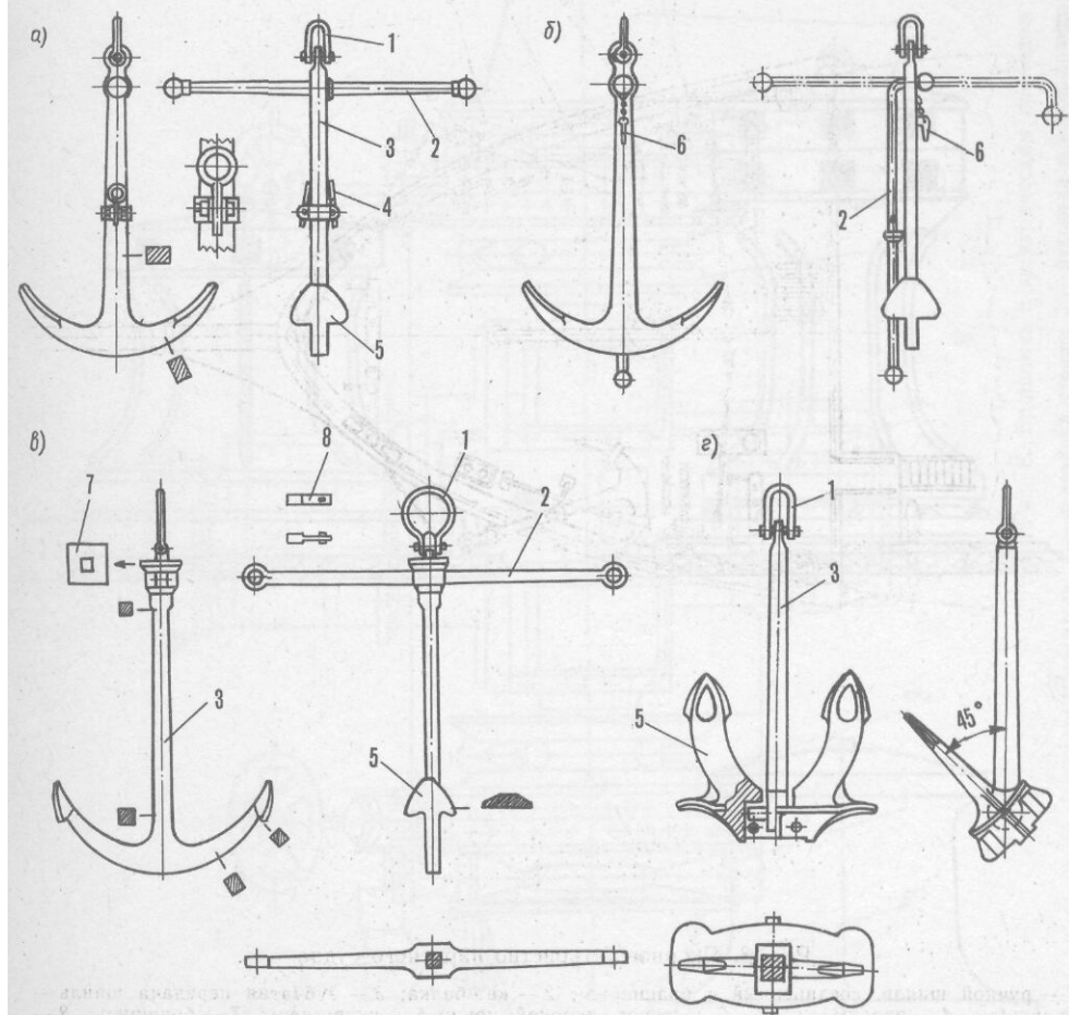
Рис. 5. Типы якорей: адмиралтейский (а, б); Роджерса (в); Холла (г) / — скоба якоря; 2 — шток; 3 — веретено; 4 — скобы для уборки якоря по-походному; 5 — рога якоря; 6, 8 — стопорные чеки; 7 — квадратная планка, запираемая чекой
