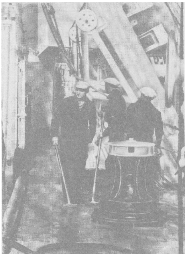
Рис. 71. Шкотовый шпиль
