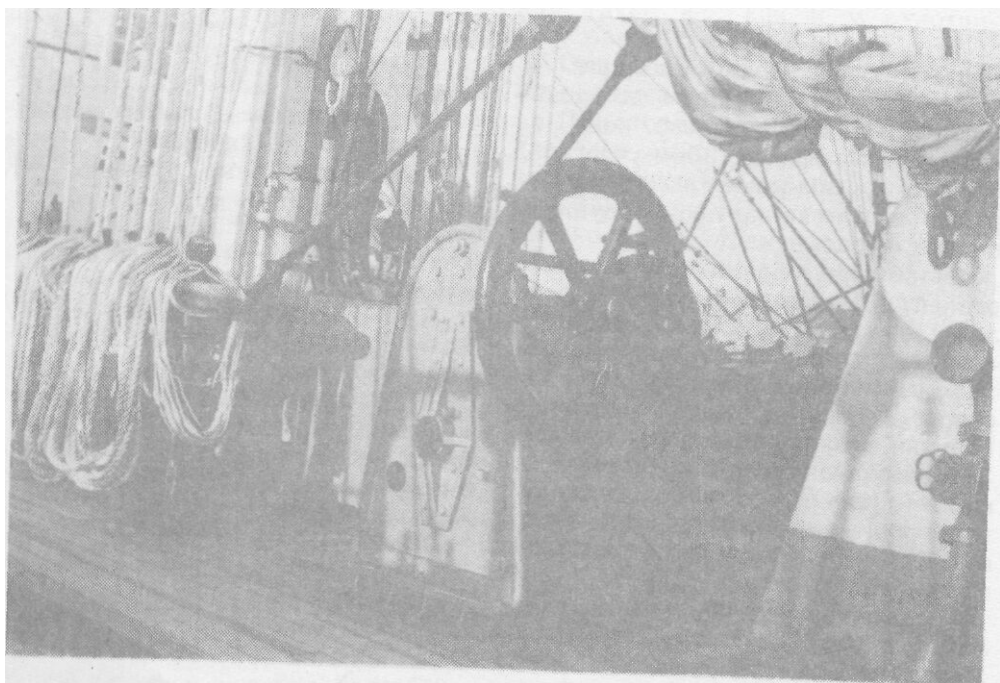
Рис. 66. Марсафальная лебедка
