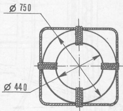
Рис. 20. Спасательный круг
