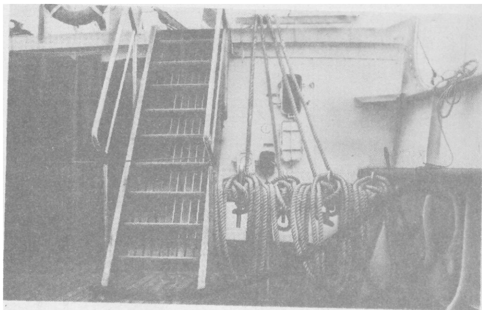
Рис. 50. Трап на полубак
