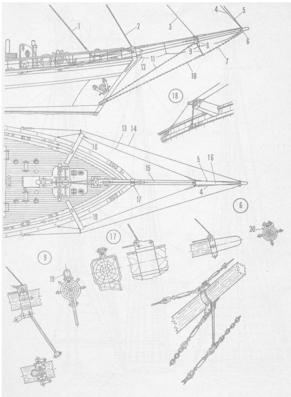
Рис. 31. Деревянный бушприт
