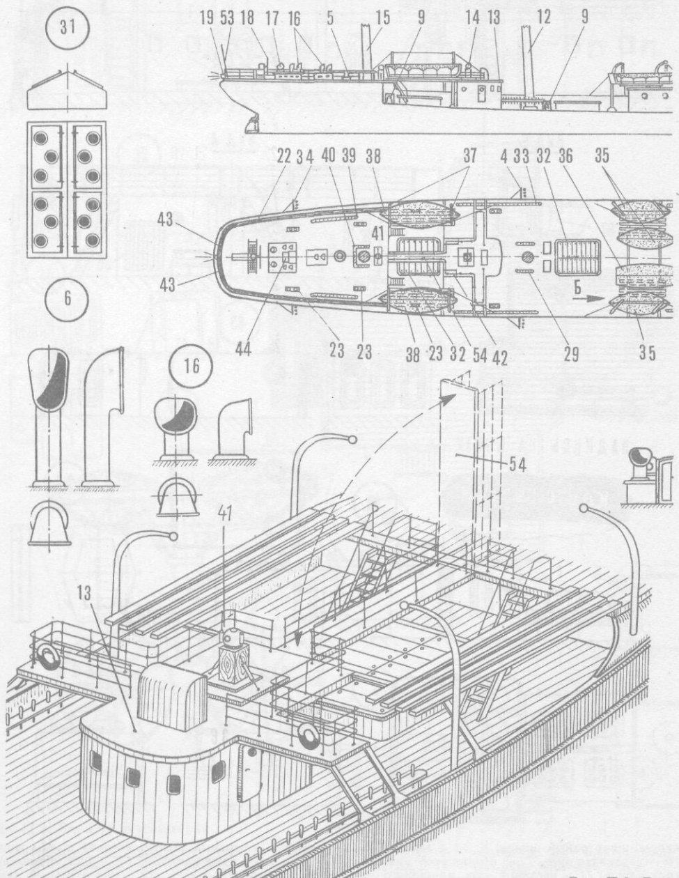
Рис. П.3. Барк
