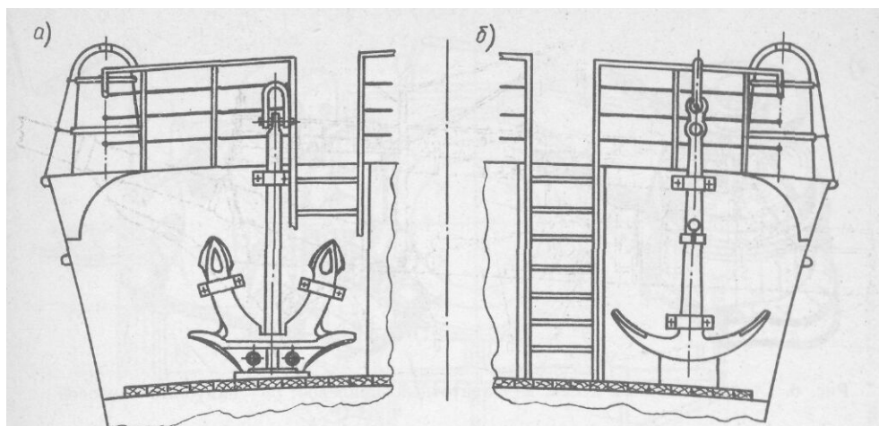
Рис. 4. Крепление запасных якорей на баке судна: а — якорь Холла; б — якорь адмиралтейский (стоп-анкер)
