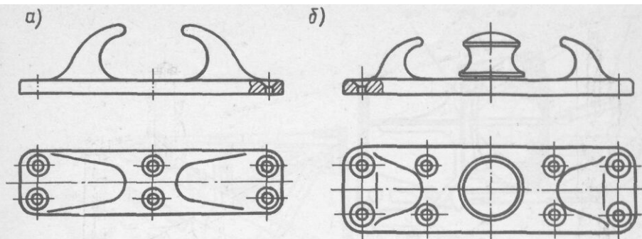
Рис. 11. Типы киповых планок: а — открытая киповая планка; б — открытая киповая планка с одним роульсом
