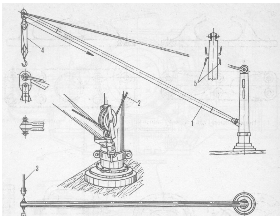
Рис. 9. Кат-балка
