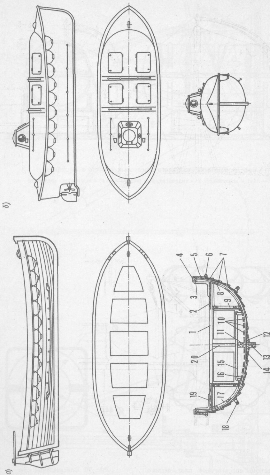
Рис. 21. Конструкция спасательной шлюпки; а — деревянной класса 1А; б — пластмассовой закрытого типа
