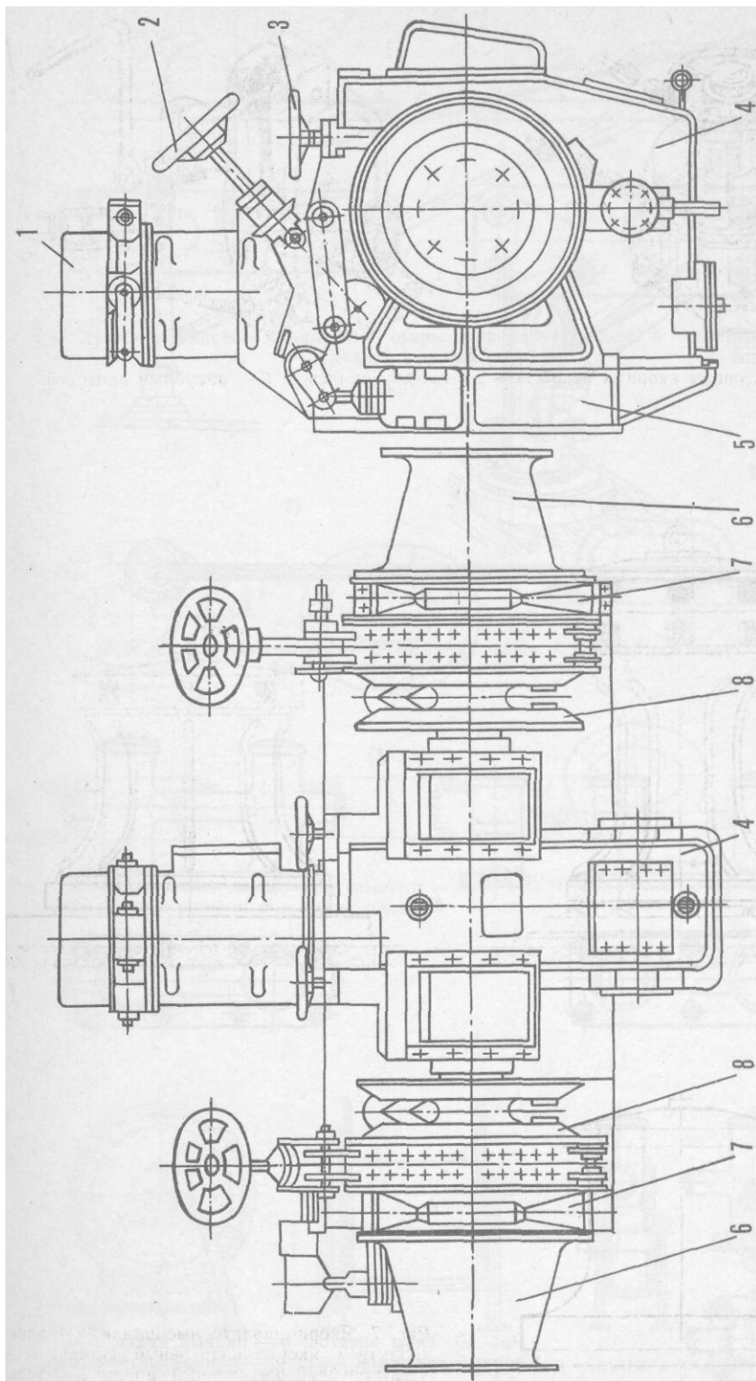
Рис. 8. Брашиль с электрическим приводом
