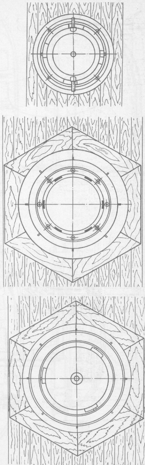
Рис. 23. Шкотовые шпиль: а — односкоростной; б — двухскоростной; в — двухскоростной дифференциальный; г — дромед; 1 — шпиль-гат; 2 — вельсы; 4 — паллед; 5 — палгун; 6 — пал; 7 — пал; 8 — съемная рукоятка
