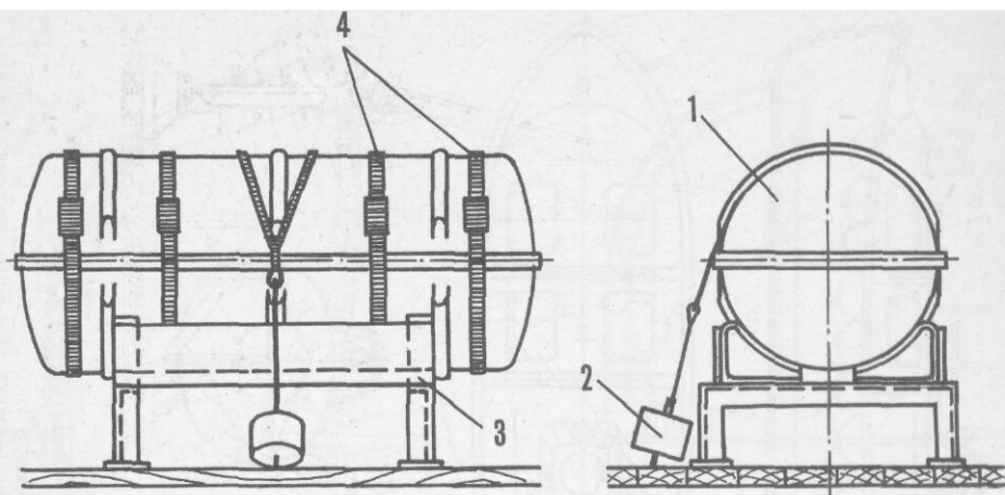
Рис. 18. Крепление надувного спасательного плота в контейнере 1 — плот в контейнере; 2 — гидростат; 3 — роостры плота; 4 — стопоры крепления
